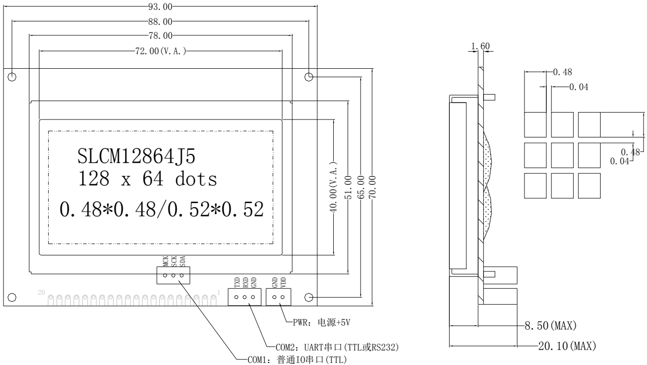
SLCM12864J3,SLCM12864J5（尺寸为：93*70）
